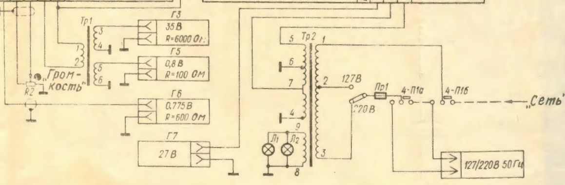
Рис. 13. Электрическая схема.
